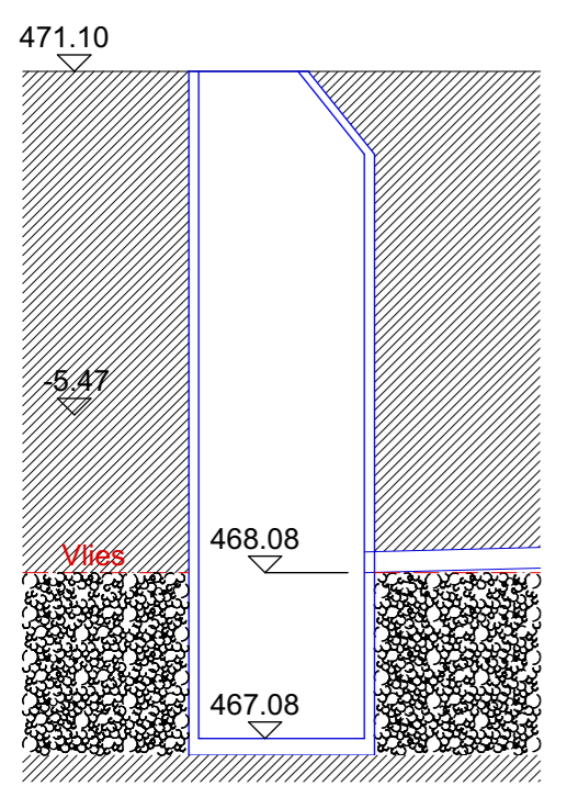
max. Grundwasserspiegel 460.96 (05.01.13) SCHNITT SICKERSCHACHT 1:50
